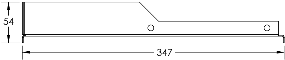
Vista lateral
